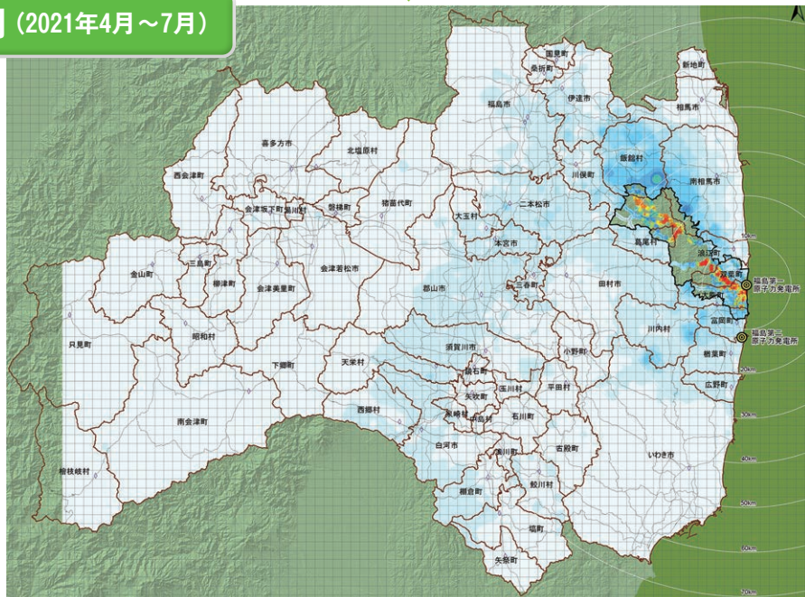
国土地理院「基盤地図情報数値標高モデル」、国土交通省国土政策局「国土数値情報(行政区域、道路)」を使用し作成。 ※帰還困難区域で実施した走行サーベイ(令和3年8月29日～10月3日実施)の測定結果を追加。
